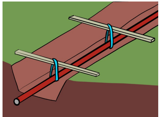
Figur 4: Ophængning af kabler med stropper på min. 5 cm bredde og for hver 1-2 meter. Kablet må aldrig hænge over længere stræk i egen vægt. Kablet beskyttes mekanisk med klikrør eller douglasplader hvis der arbejdes tæt ved kablet når det er frigravet
